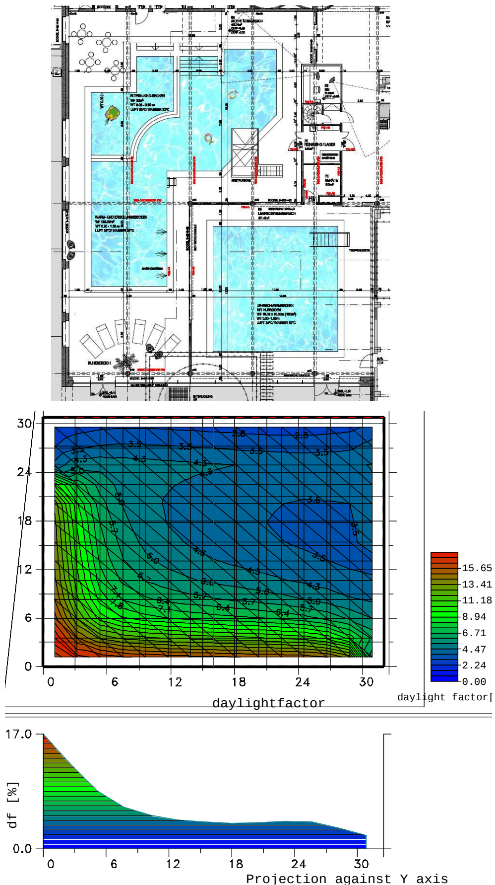
Abbildung 33: Tageslichtkoeffizient für den Hallenabschnitt Süd-West
