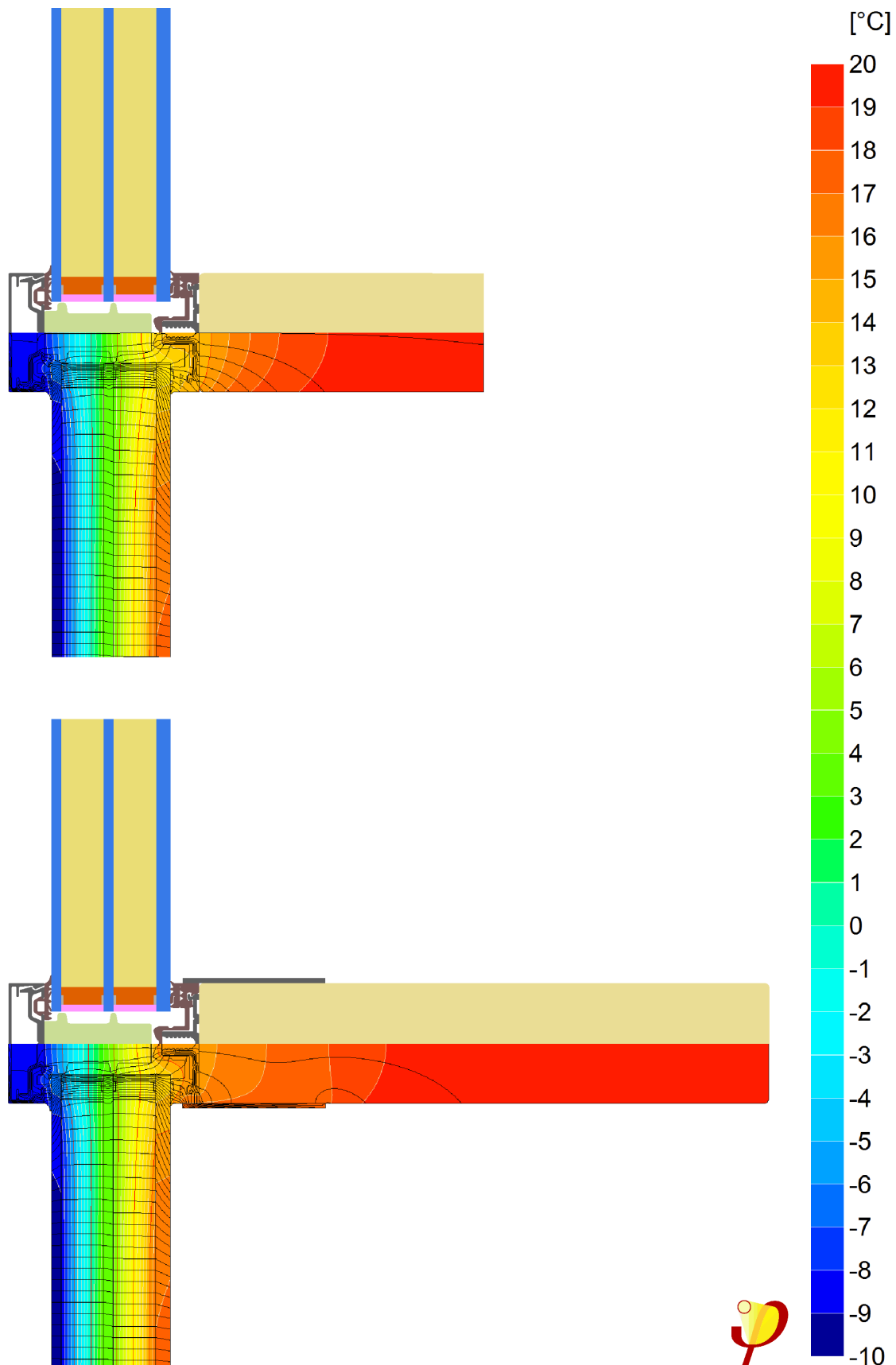
Abbildung 15: Pfosten-Riegel-Fassade Raico Therm+ 50 h-v in den im Lippebad verwendeten Versionen (Oben: Berechnungsmodell, unten: Isothermengrafik mit Temperatur- und Wärmestromlinien). In der Halle wird eine Variante mit Wärmeleitblechen zur Erhöhung der Glasrandtemperatur zur Anwendung kommen (untere Abbildung) (Quelle: PHI)
