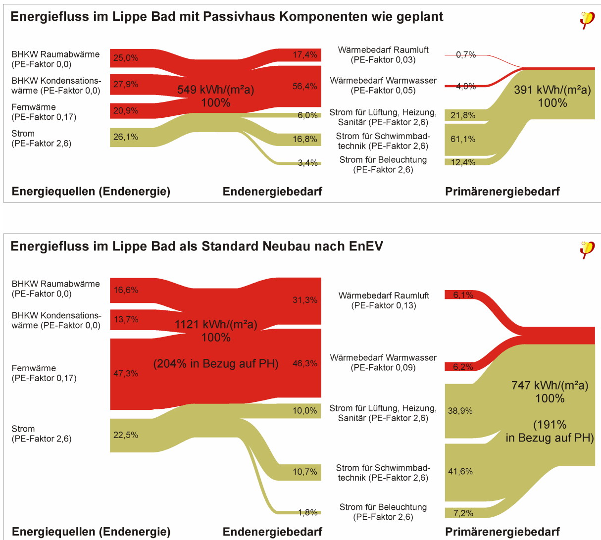
Abbildung 54: Grafische Darstellung des Energiebedarfes der Varianten PH und EnEV
