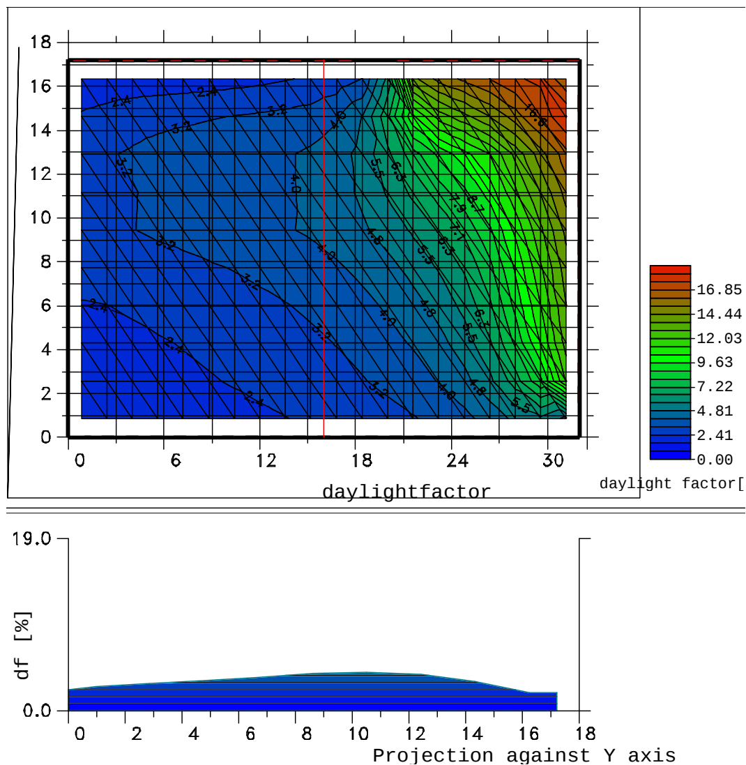
Abbildung 32: Tageslichtkoeffizient für den Hallenabschnitt Ost mit optimierten Fensterflächen
