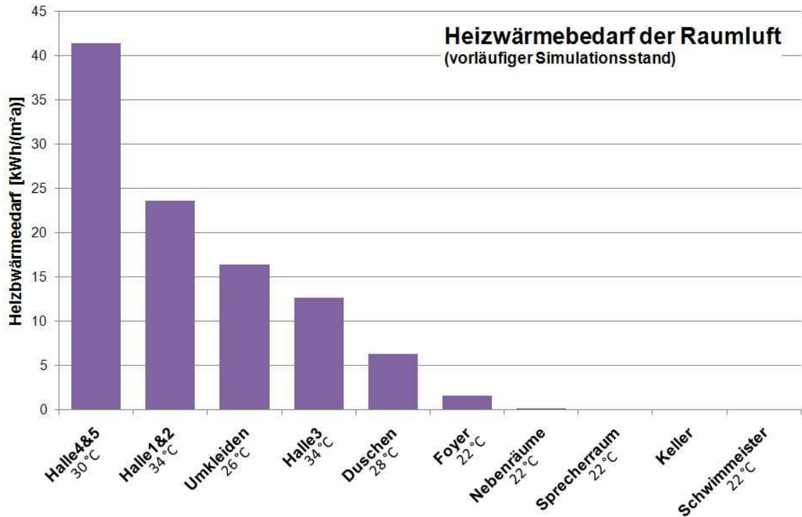
Abbildung 48: Der mit der dynamischen Simulation berechnete Heizwärmebedarf der Raumlufth, absteigend sortiert.
