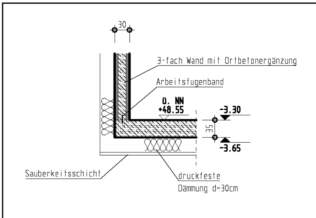
Abbildung 14: Systemdetail Übergang Sohle-Wand (Quelle: Ostermann)
