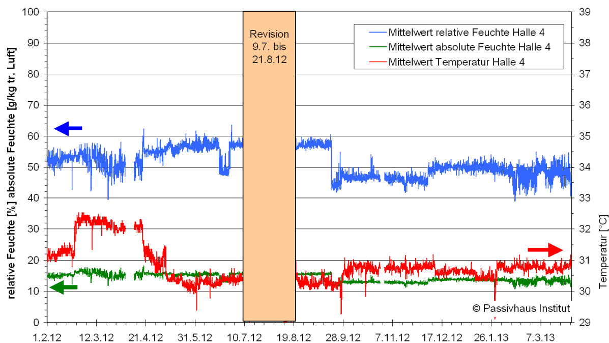
Abbildung 45: Verlauf der mittleren Hallentemperatur, der relativen sowie absoluten Feuchte in Halle 4 vom 01.02.2012 bis zum 01.04.2013 (Stundendaten)
