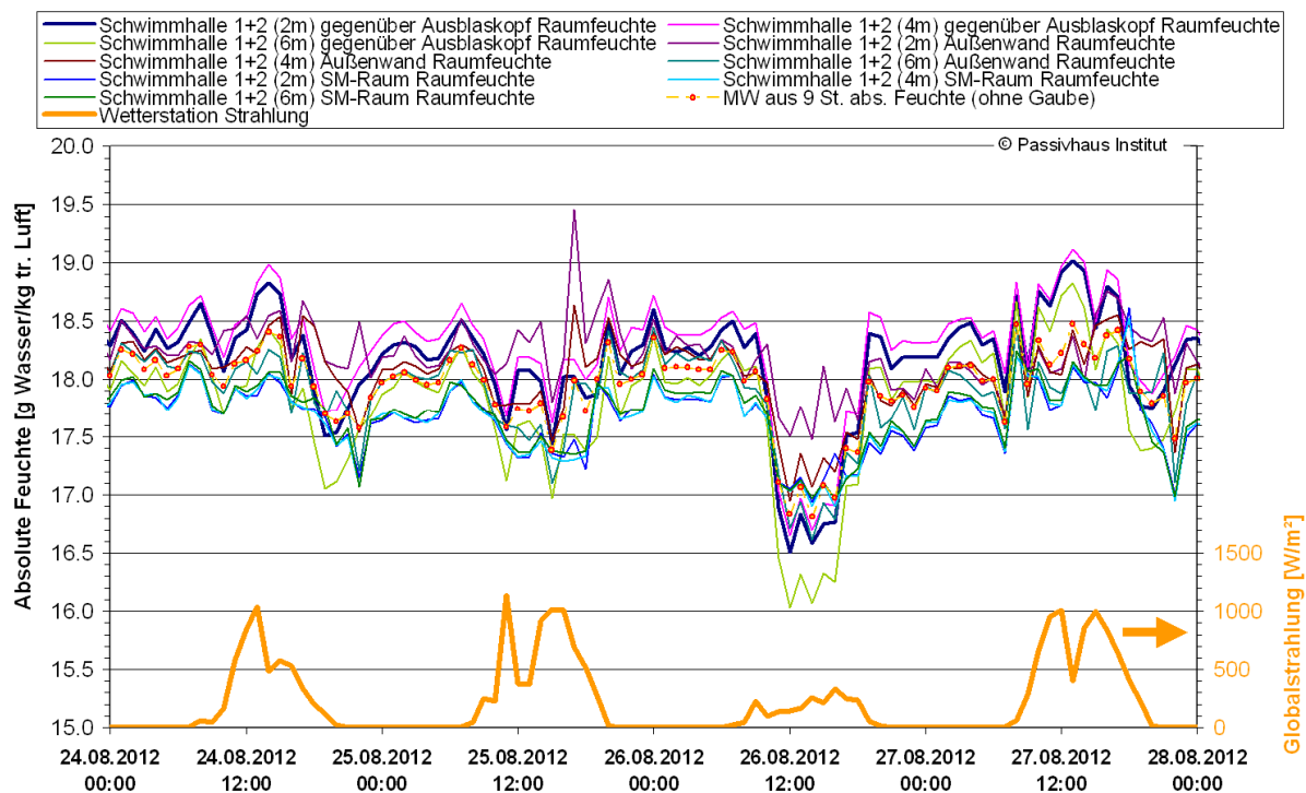
Abbildung 30: Absolute Raumlufffeuchten der neun Sensoren in Halle 1+2 und die „mittlere absolute Hallenfeuchte“ (siehe Text) sowie die Globalstrahlung vom 24. bis zum 27. August 2012 (Stundenmittelwerte).
