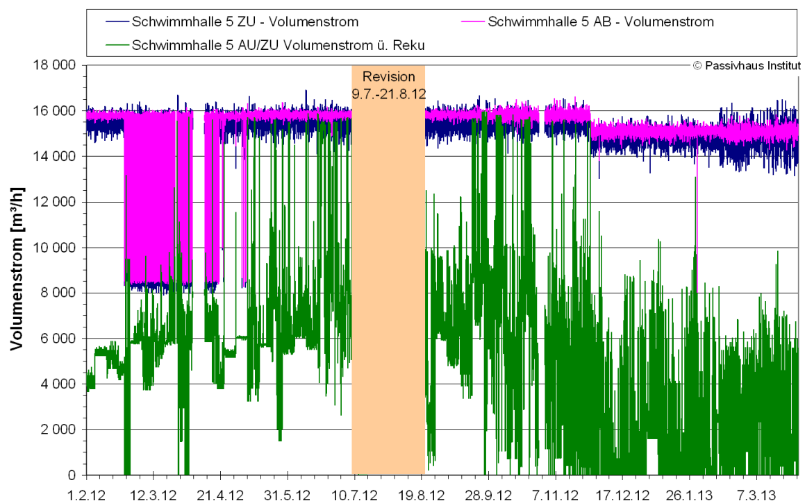
Abbildung 58: Volumenströme der Lüftungsanlagen von Halle 4 und 5 vom 01.02.2012 bis zum 31.3.2013 (Tageswerte)
