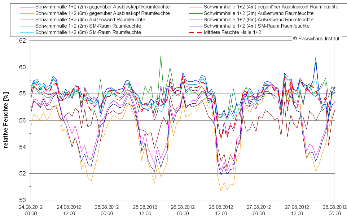
Abbildung 29: Relative Raumlufffeuchten der neun Sensoren in Halle 1+2 und die „mittlere rel. Hallenfeuchte“ (siehe Text) vom 24. bis zum 27. August 2012 (Stundenmittelwerte).
